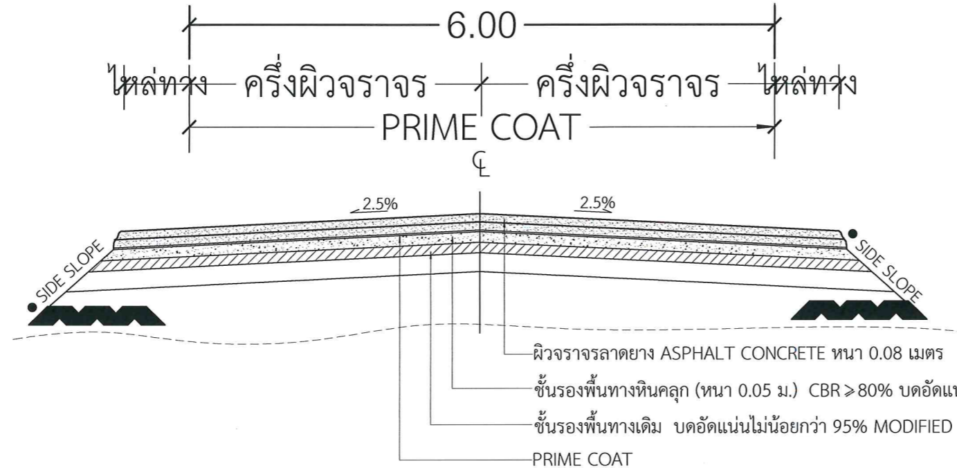
รูปตัดแสดงโครงสร้างถนน
